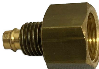
COD.189 CONEXÃO SAÍDA DE AR ROSCA INTERNA M16 X 1,5 IVECO /VOLVO
