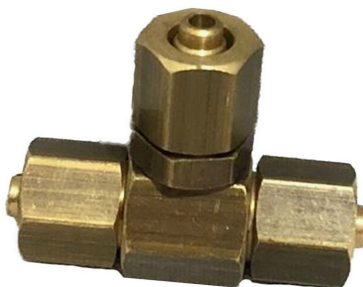
COD.198 TEE DE REDE 1/4 C/ BICO 1/4
